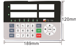
正视图 Front view
